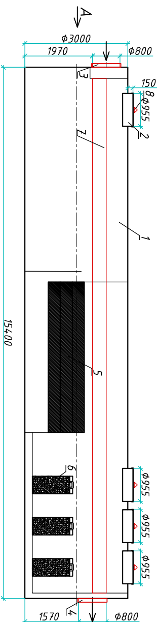
Разрез 1-1
