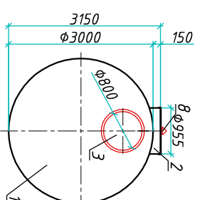
Вид А
