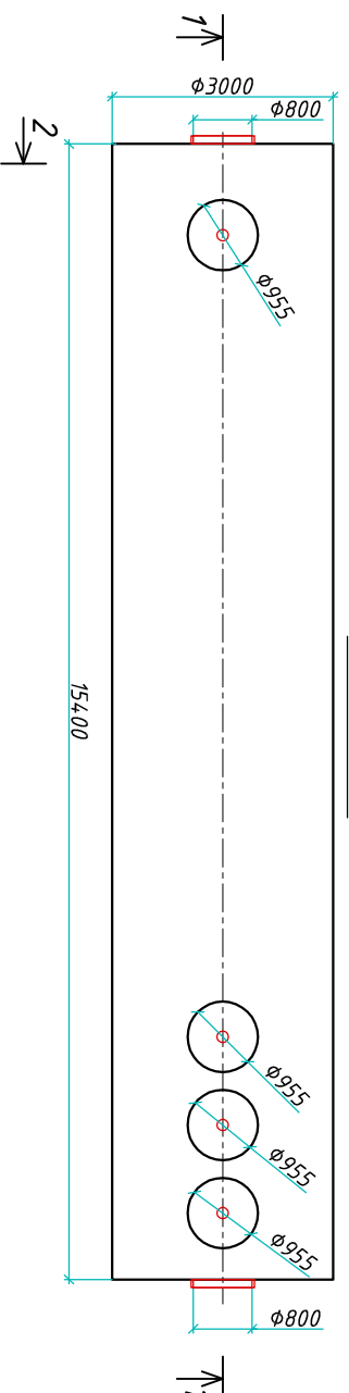
Вид сверху
